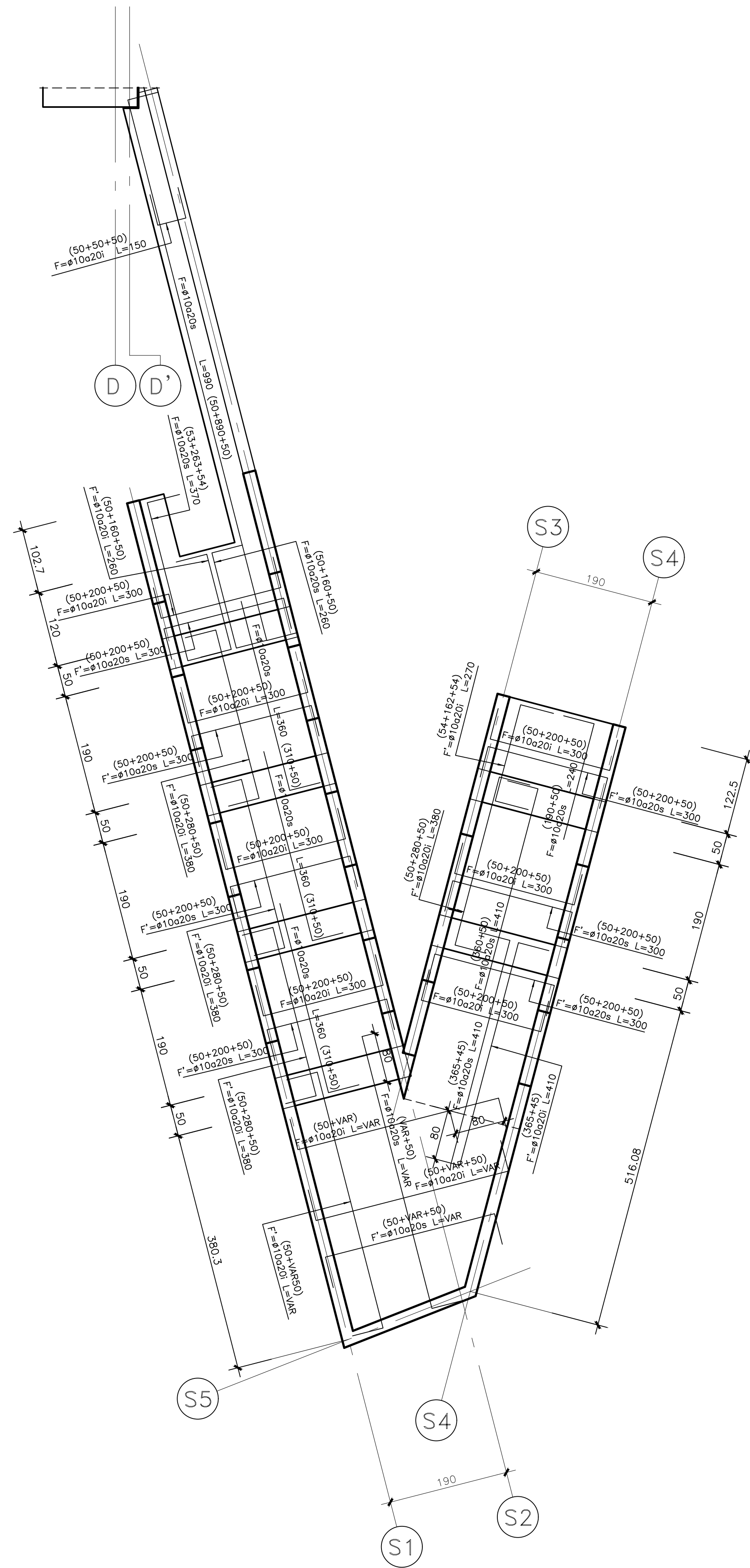
PLANTA ARMADURA DE FUDACION ESCALERA 03 EXTERIOR SUR
