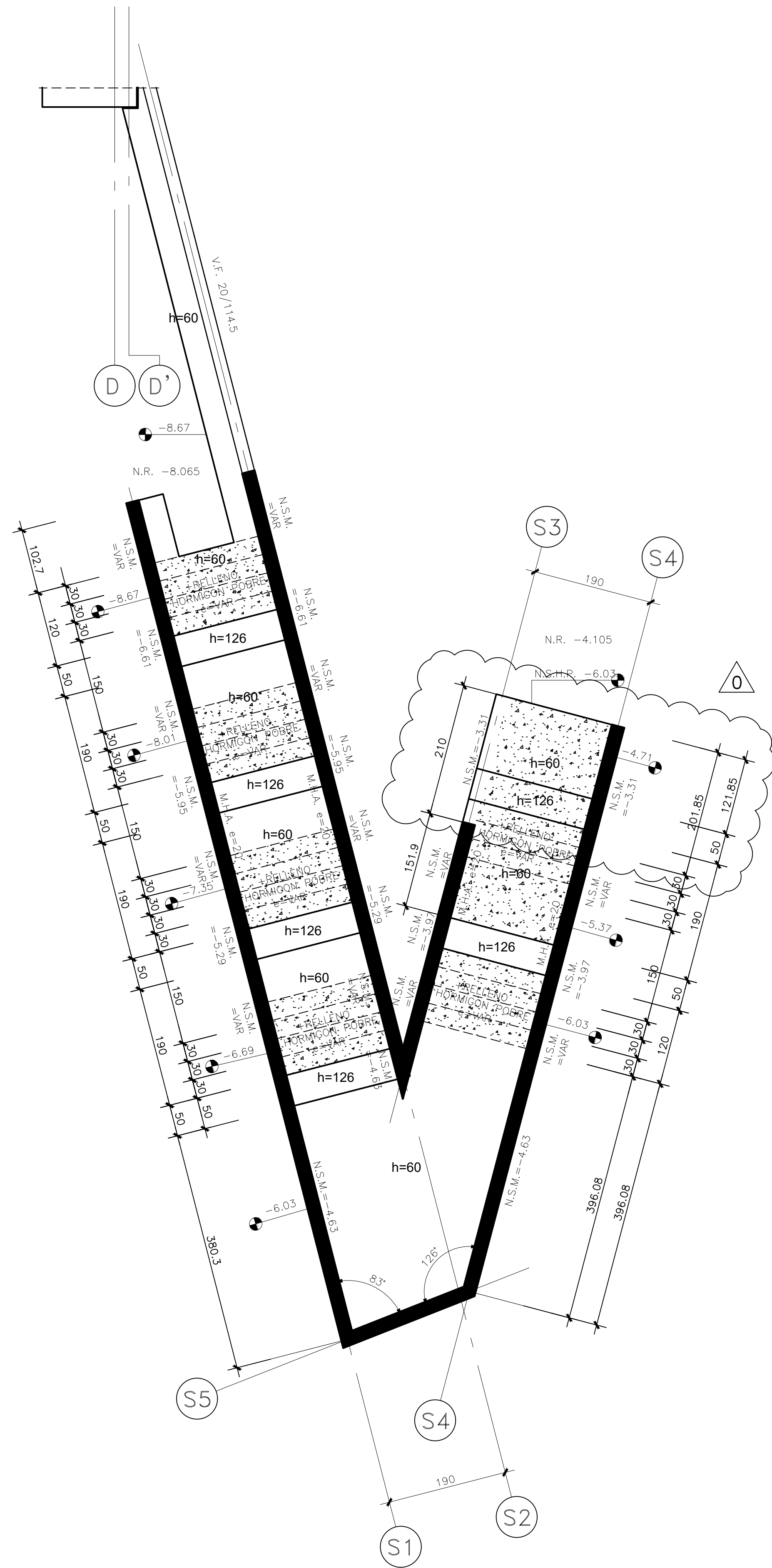
PLANTA ESCALERA 03 EXTERIOR SUR DESDE NIVEL -8.065 al -4.105
